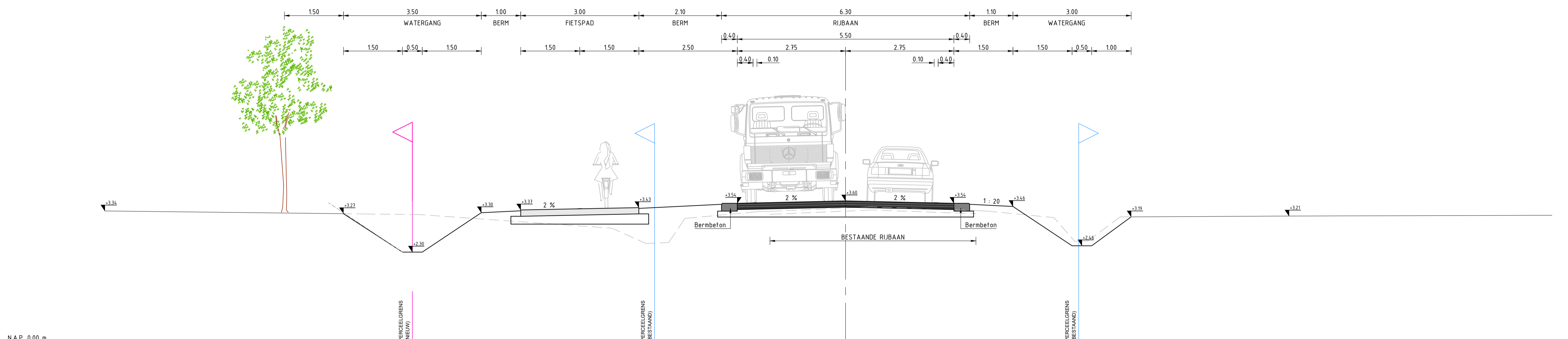
Profiel J-J 1:50
