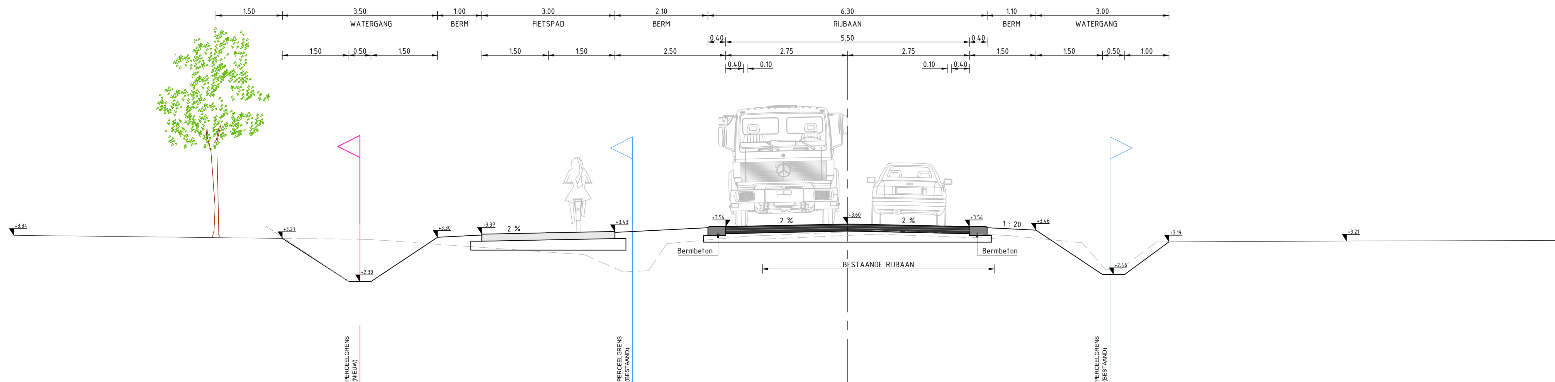
Profiel J-J 1:50
