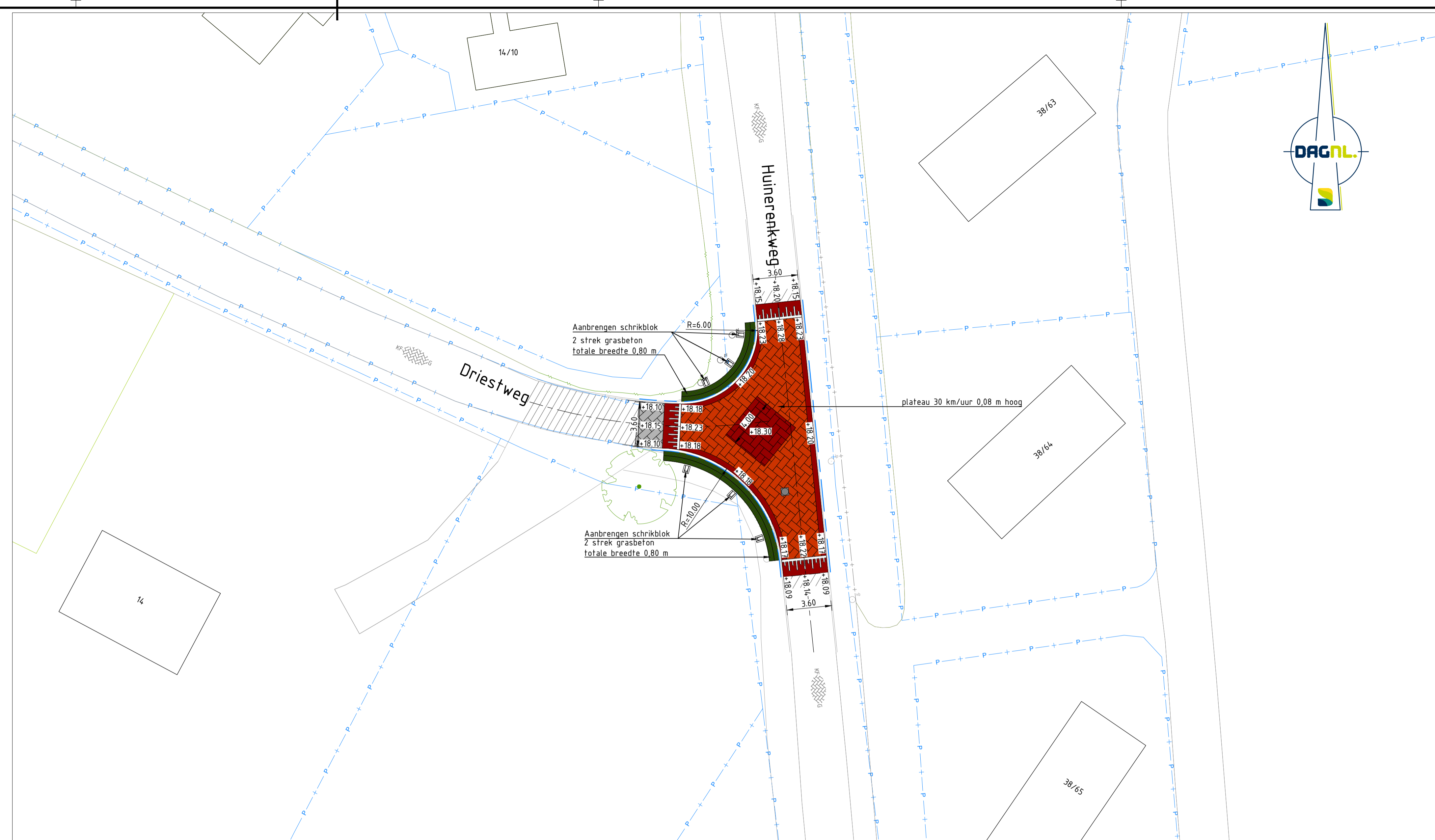
SITUATIE 3.2 schaal 1:200
