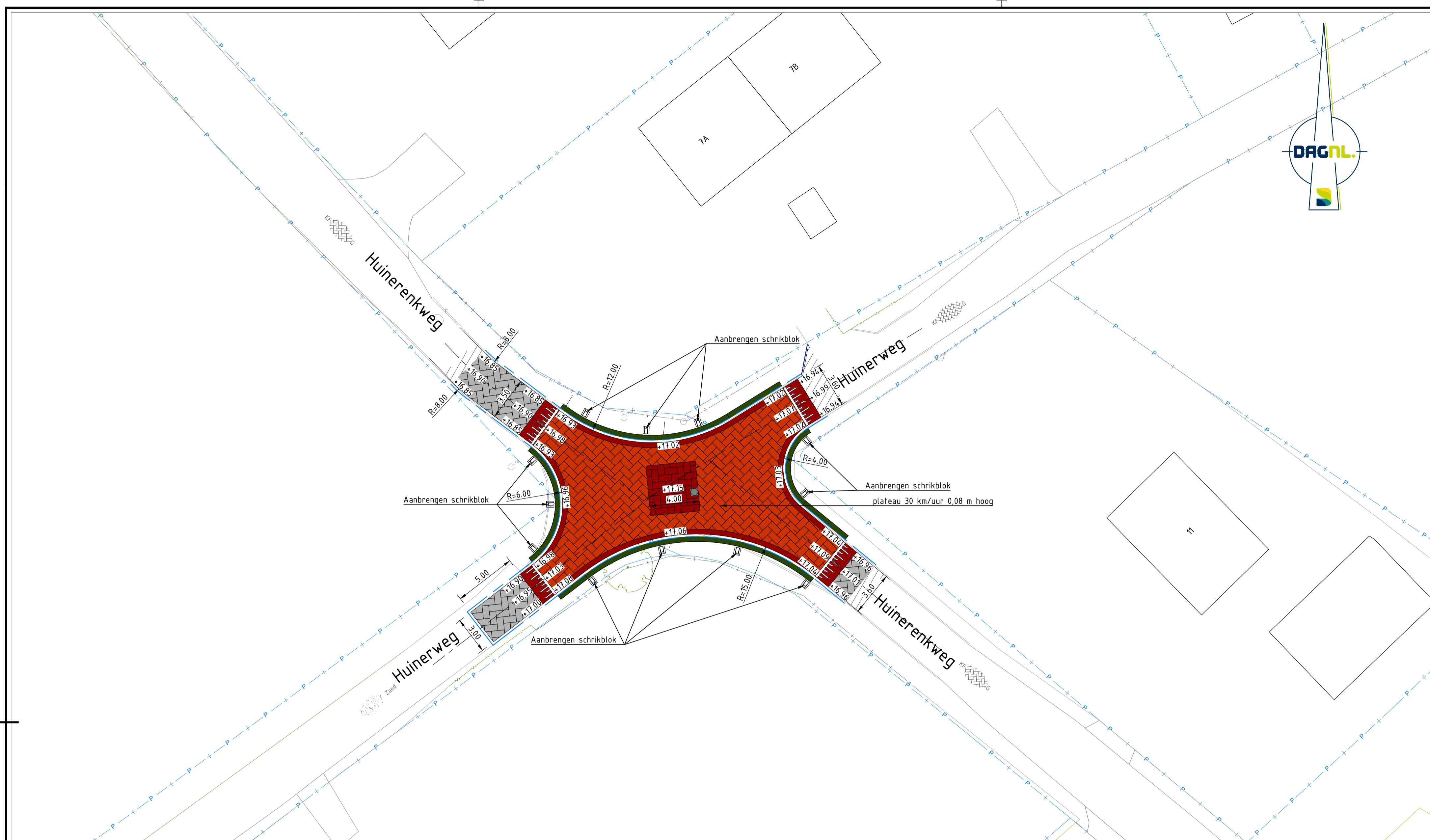
SITUATIE 3.1 schaal 1:200
