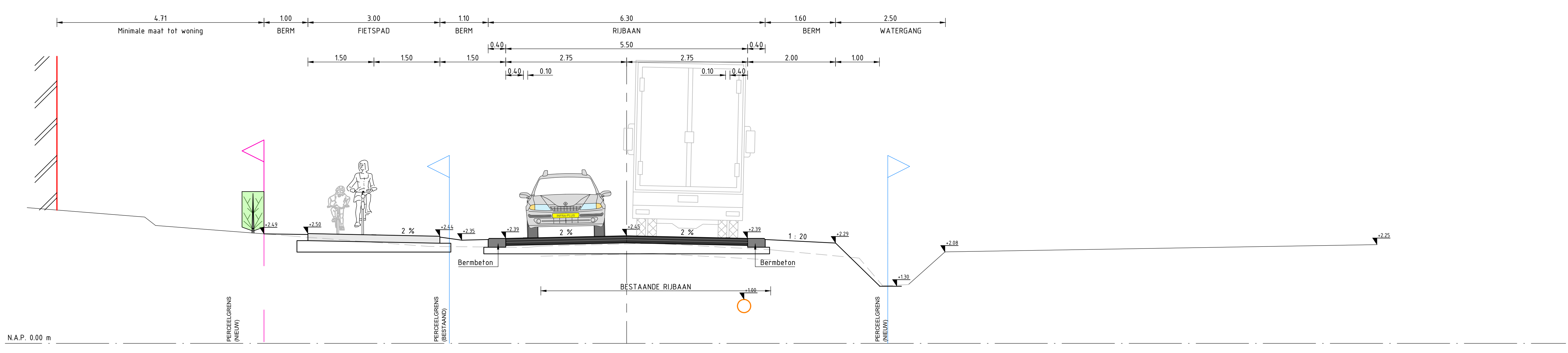
Profiel A'-A' 1:50
